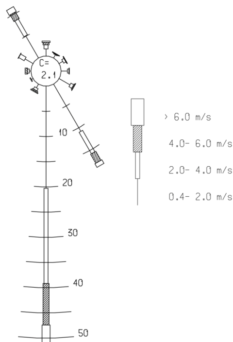
Figur 6: Vindrosen fra Svanvik og Karpdalen for periodene april-september 2011 og oktober 2011-mars 2012 (vindrosene viser frekvensen av vind i tolv 30-graders sektorer, dvs. hvor ofte det blåser fra disse retningene).
