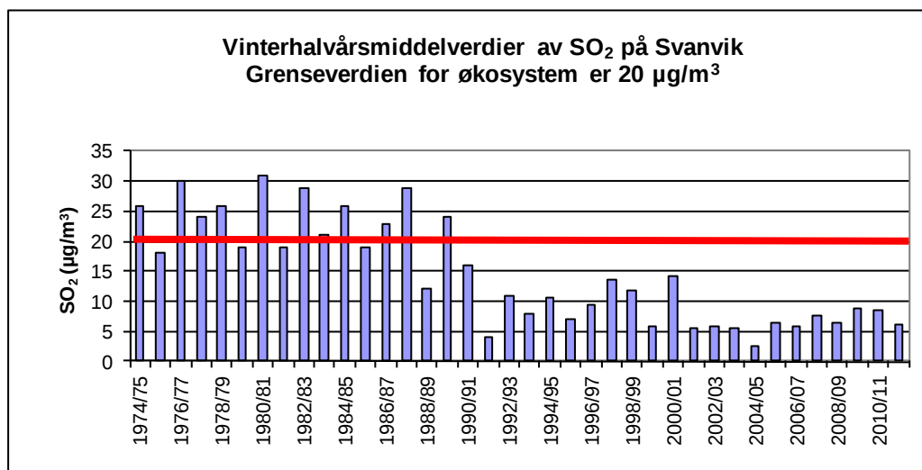
Figur 21: Vinterhalvårsmiddelverdier av SO 2 på Svanvik 1974/75-2011/12 (enhet: µg/m 3 ).
