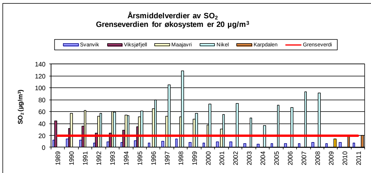
Figur 20: Årsmiddelverdier av SO 2 på Svanvik (1989-2011), på Viksjøfjell (1989-1995), i Maajärvi (1990-2001), i Nikel (1992-2008) og i Karpdalen (2009-2011) (enhet: µg/m 3 ).
