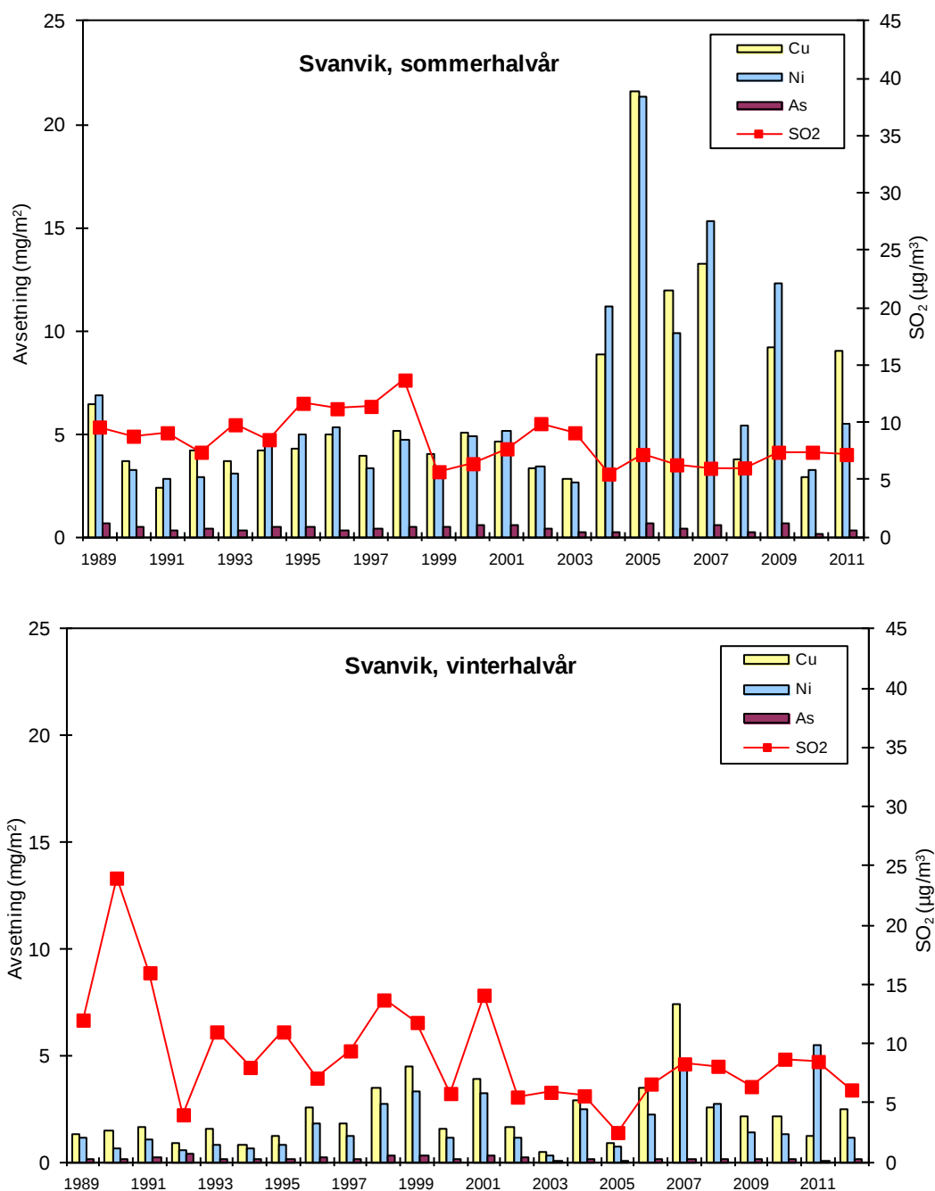
Figur 24: Avsetning med nedbør av Cu, Ni og As (mg/m 2 ) i sommerhalvårene fra 1989 til 2011 og i vinterhalvårene fra 1988/89 til 2011/12. Halvårsmiddelkonsentrasjonene av SO 2 er også vist (µg/m 3 ).
