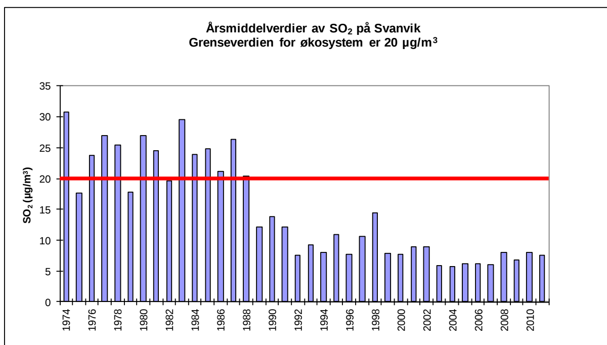
Figur 19: Årsmiddelverdier av \text{SO}_2 på Svanvik i årene 1974-2011 (enhet: \mu\text{g}/\text{m}^3 ).
