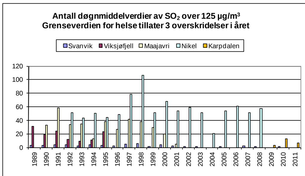
Figur 15: Antall døgnmiddelverdier av SO 2 over grenseverdien på 125 \mu\text{g}/\text{m}^3 på Svanvik (1989-2011), på Viksjøfjell (1989-1995), i Maajärvi (1990-2001), i Nikel (1992-31. august 2008) og i Karpdalen (2009-2011). Det er tillatt med 3 overskridelser i året i Norge.
