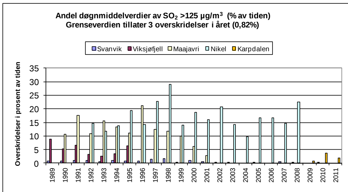
Figur 16: Andel av tiden grenseverdien for døgnmiddel av \text{SO}_2 på 125 \mu\text{g}/\text{m}^3 er overskredet på Svanvik (1989-2011), på Viksjøfjell (1989-1995), i Maajärvi (1990-2001), i Nikel (1992-31. august 2008) og i Karpdalen (2009-2011). 3 tillatte overskridelser i året tilsvarer 0,82% av tiden.
